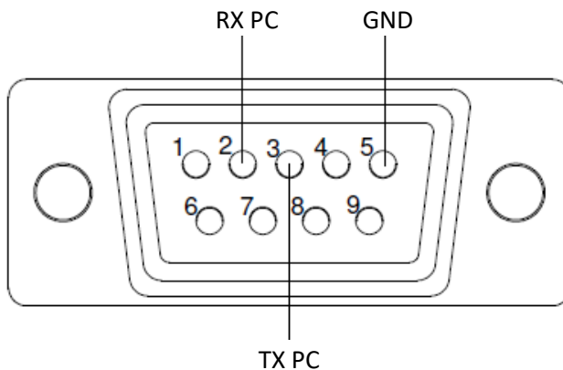
Figuur 25 : Bedrading naar DB9-connector
