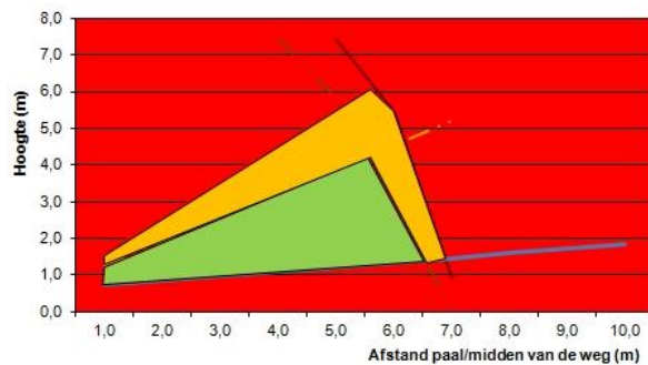
Tekening 2: twee richtingen detectie
