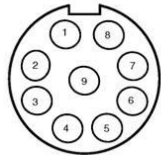
Figuur 24: TMS-SA radar-connector Weipu SP1712/P9
