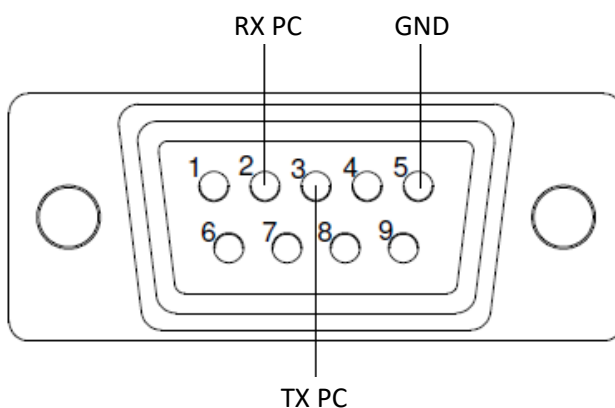
Figure 33 : brochage connecteur DB9
