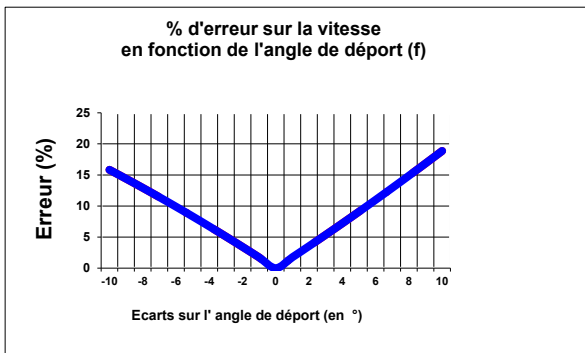
Graphique 4 : % d'erreur sur la vitesse en fonction de la variation de l'angle de déport
