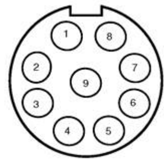
Figure 32 : connecteur Weipu SP1712/P9 du radar TMS-SA
